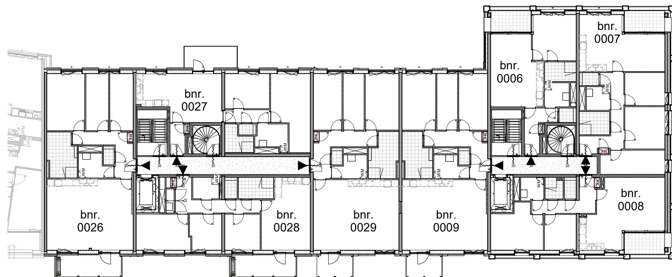
3b_2e verdieping woningoverzicht
