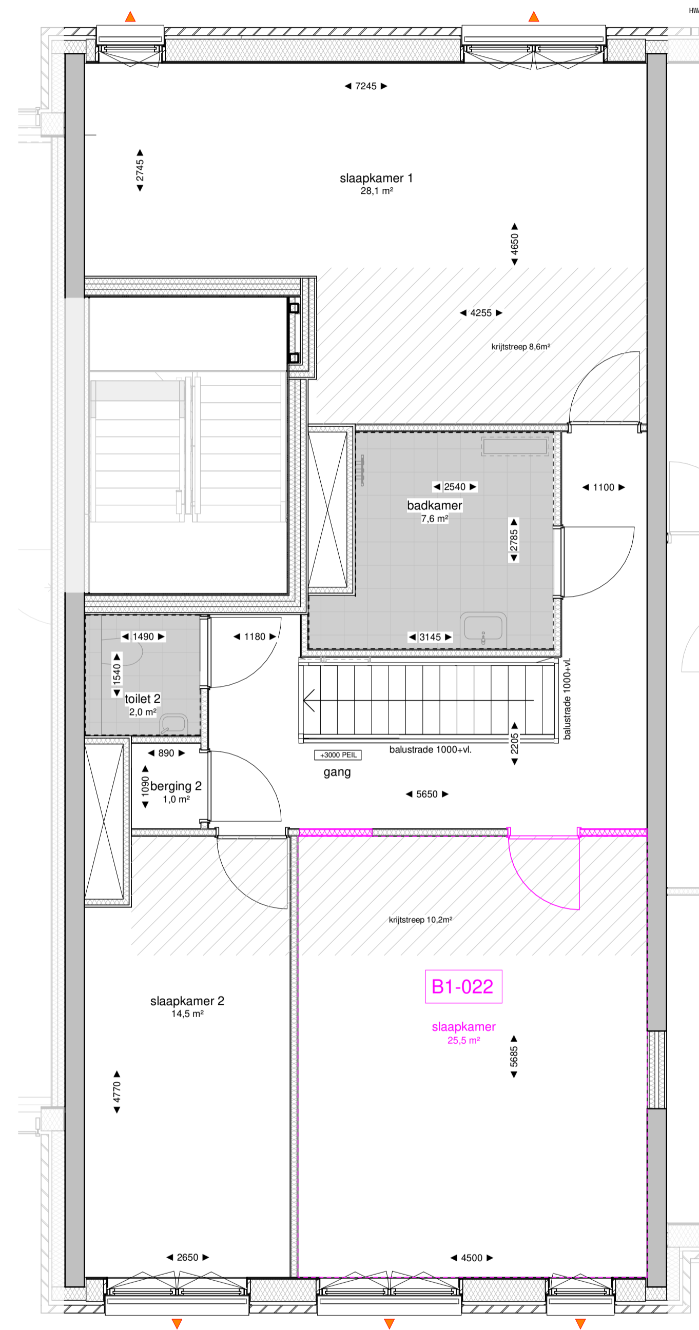
161-01 eerste verdieping optie schaal 1 : 50
