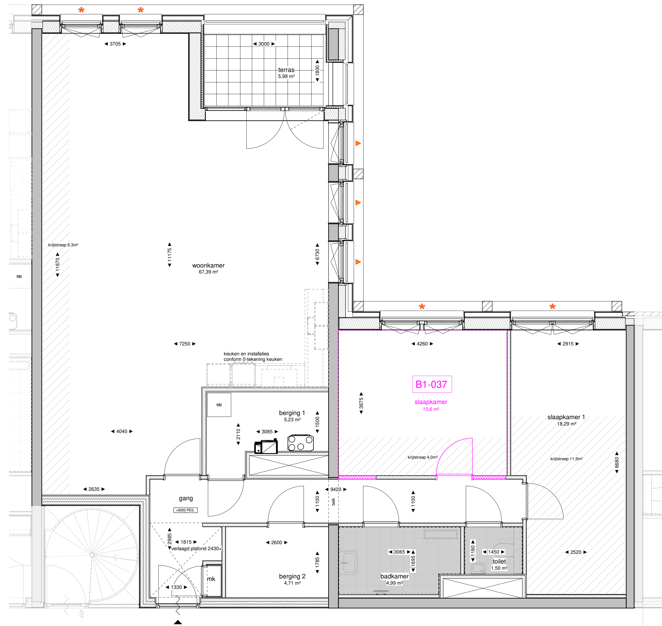
171-03 derde verdieping optie schaal 1 : 50
