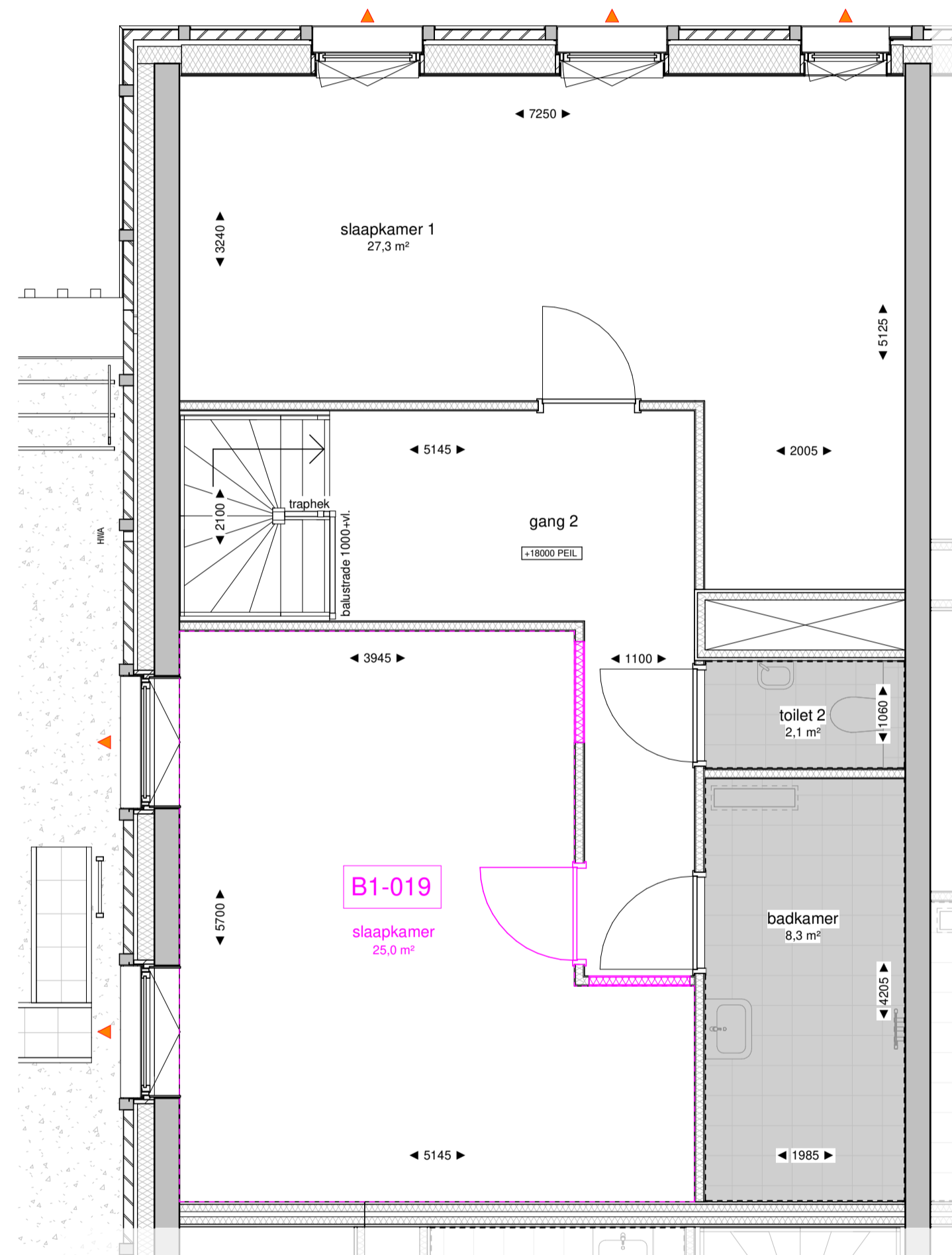
150-06 zesde verdieping optie schaal 1 : 50
