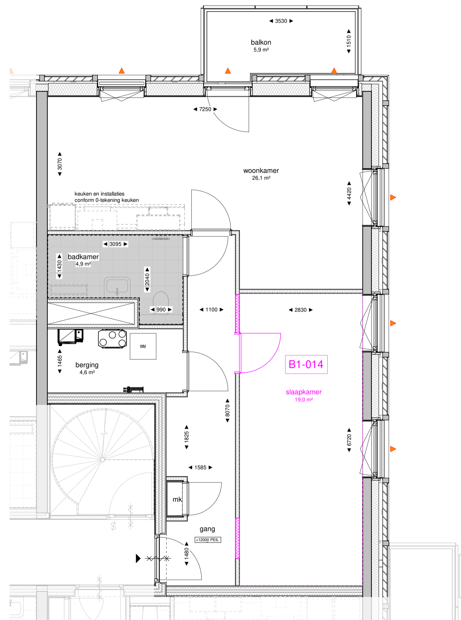
147-04 vierde verdieping optie schaal 1 : 50
