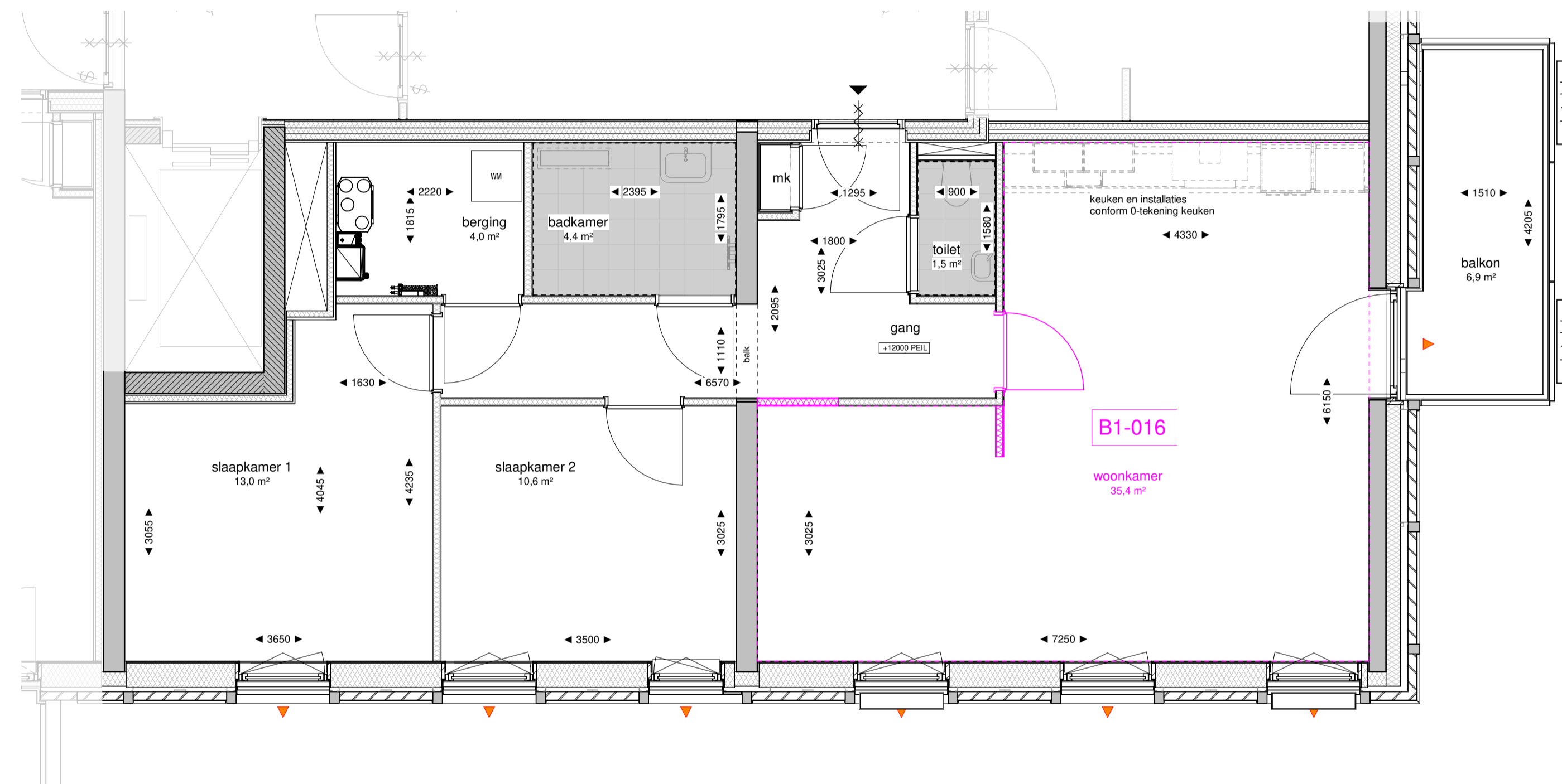
148-04 vierde verdieping optie schaal 1 : 50
