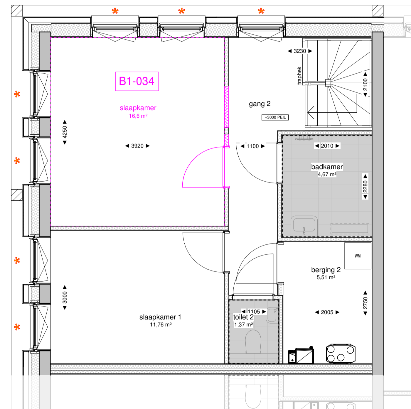
153-01 eerste verdieping optie schaal 1 : 50
