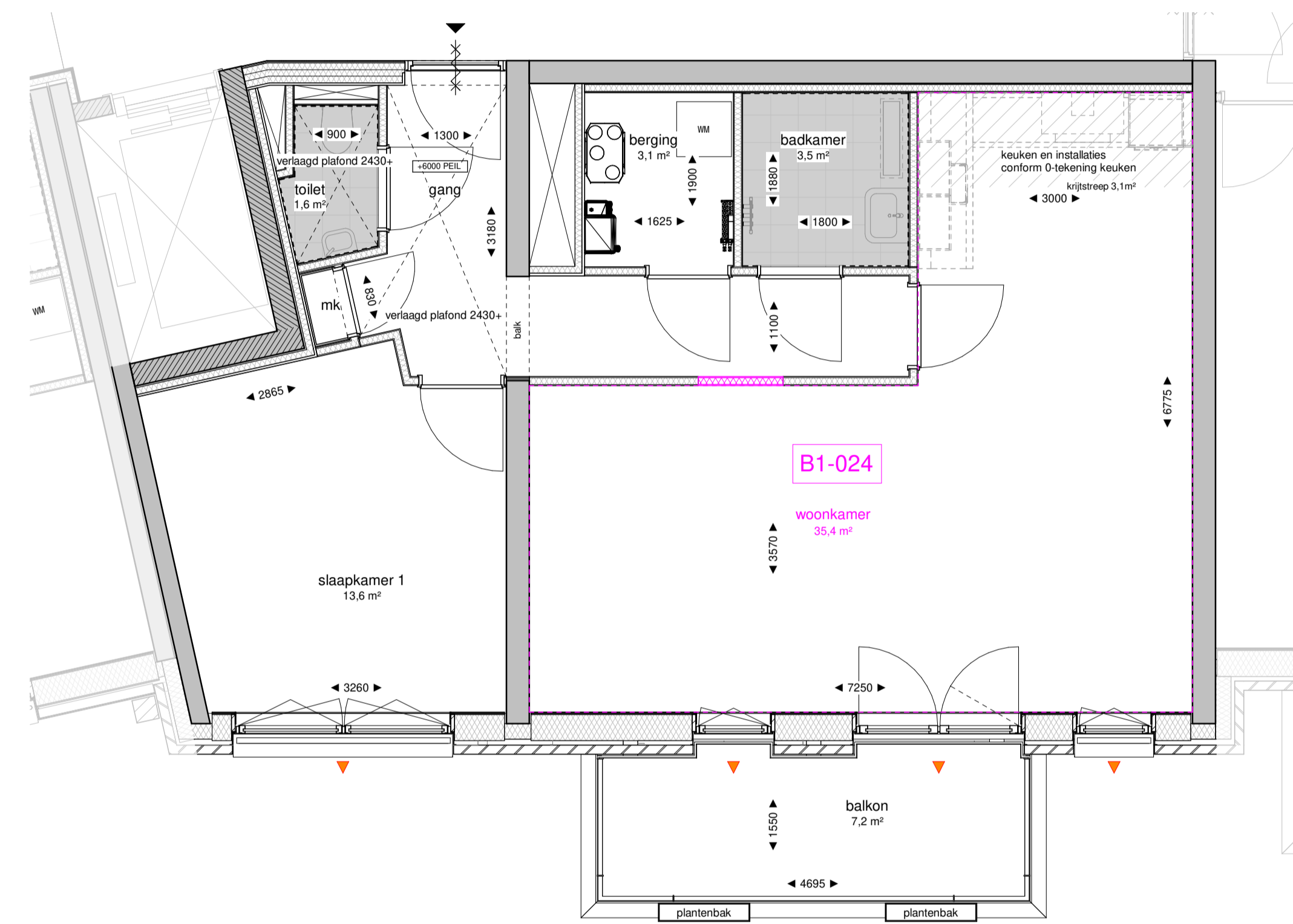
167-02 tweede verdieping optie schaal 1 : 50
