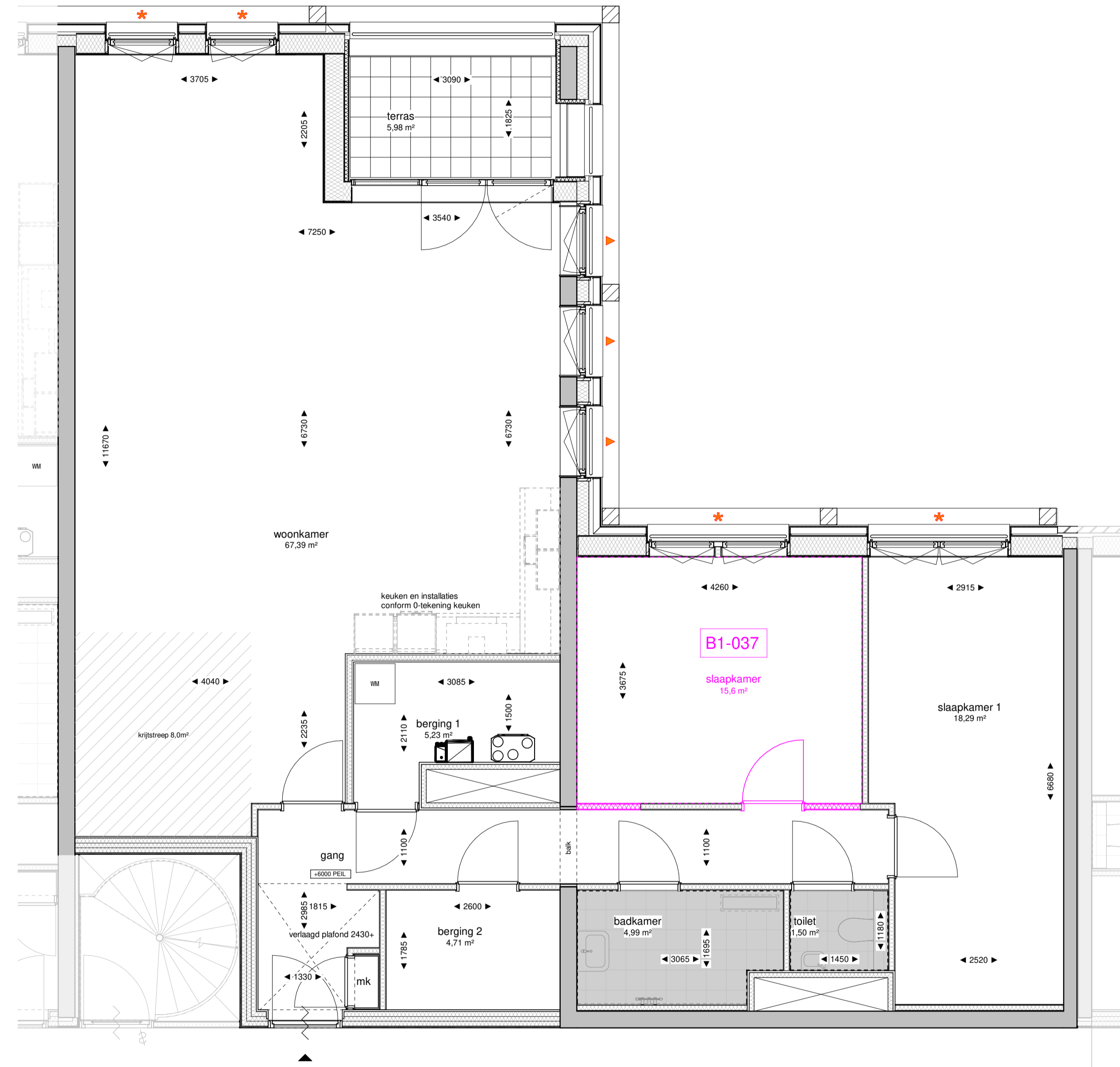
166-02 tweede verdieping optie schaal 1 : 50
