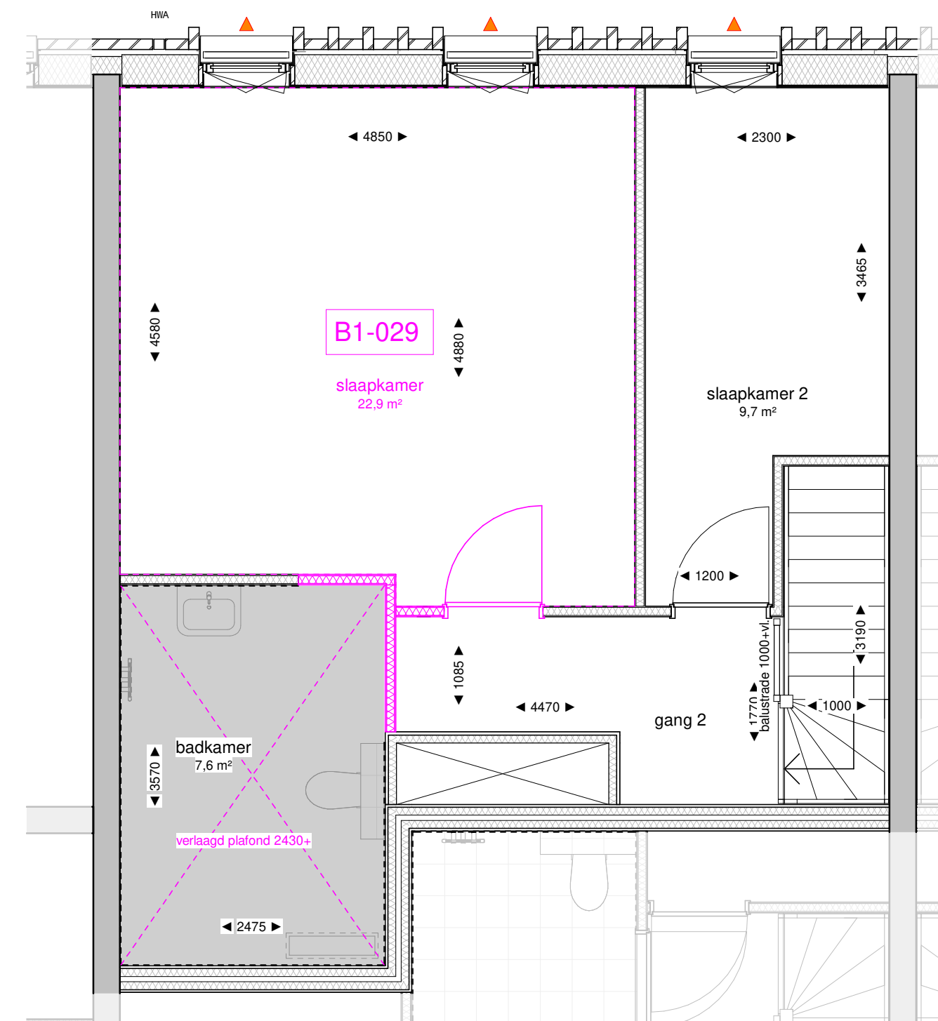
181-05 vijfde verdieping optie schaal 1 : 50
