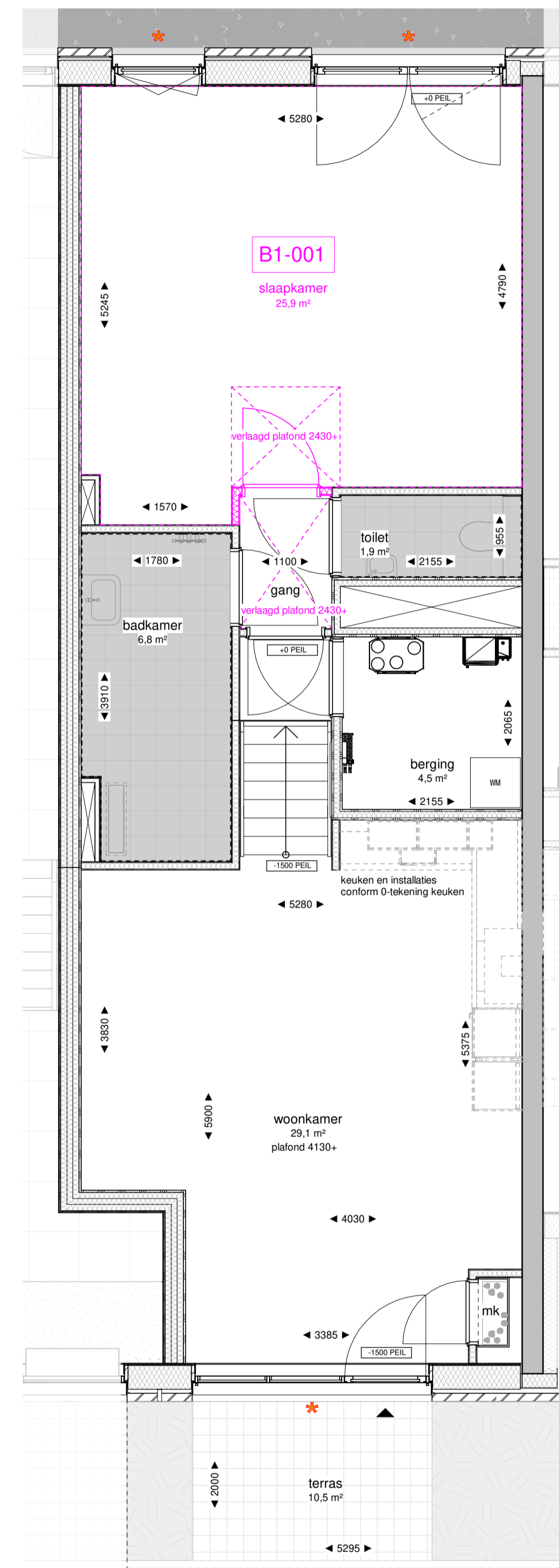
108-00 begane grond optie schaal 1 : 50
