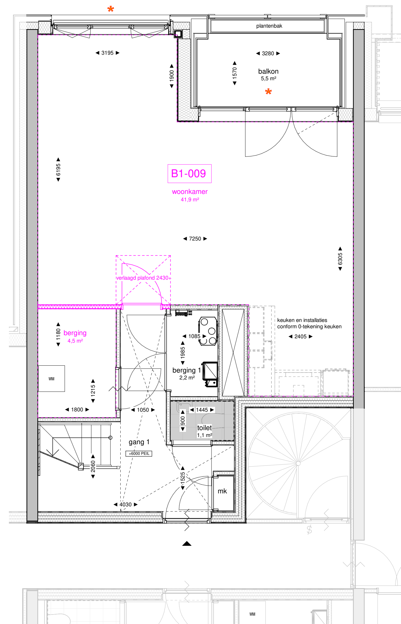
118-02 tweede verdieping optie schaal 1 : 50
