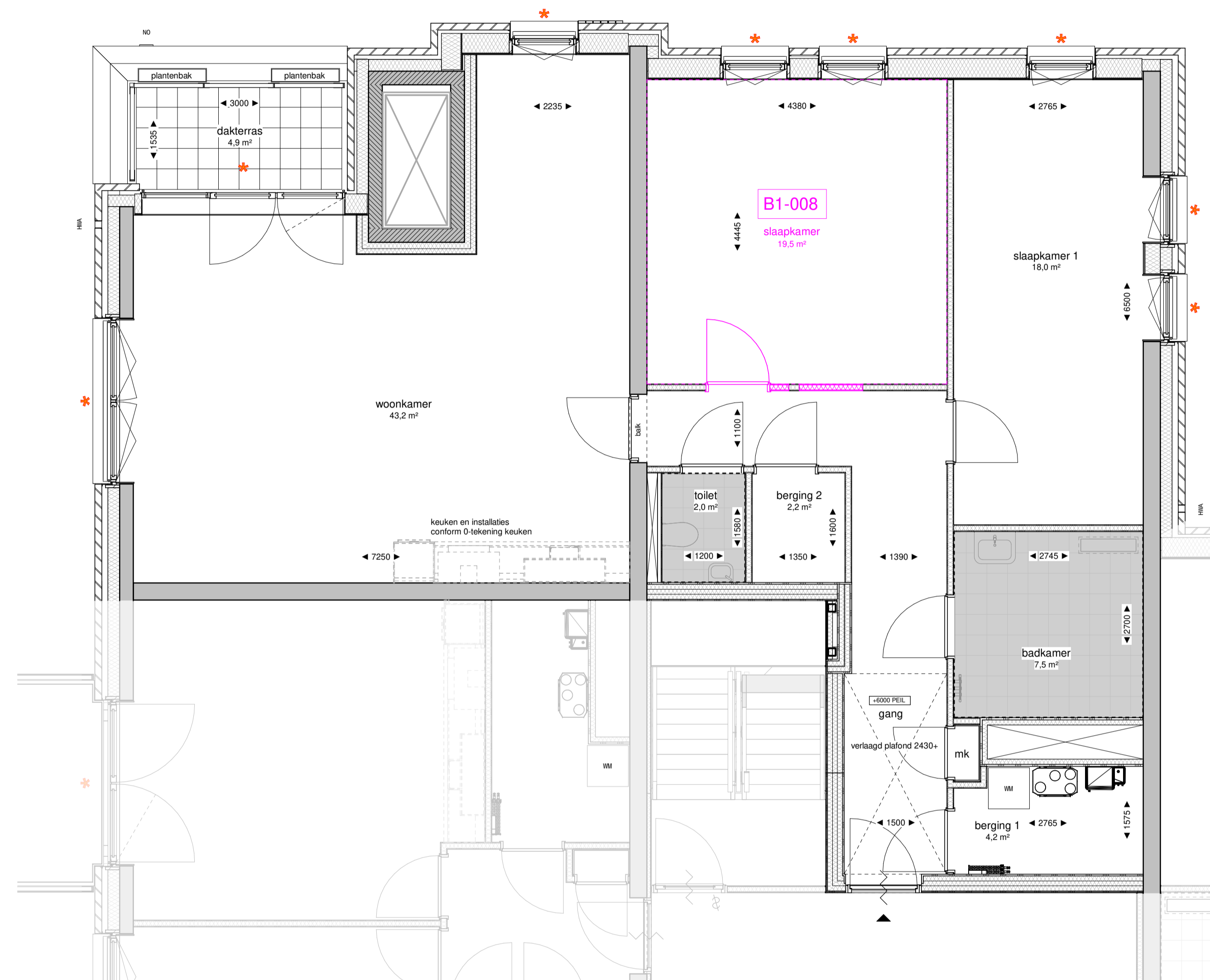
125-02 tweede verdieping optie schaal 1 : 50
