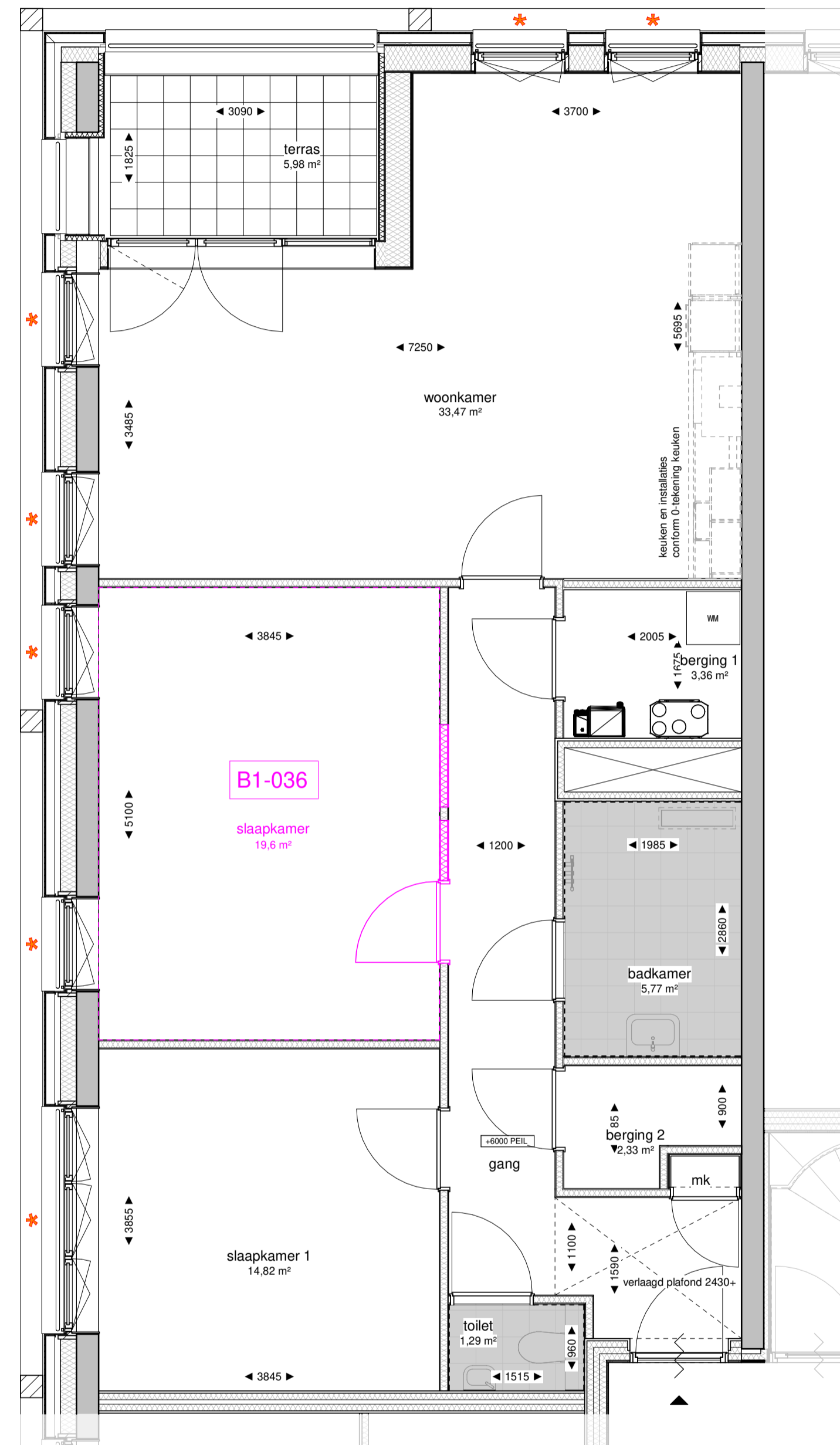
163-02 tweede verdieping optie schaal 1 : 50
