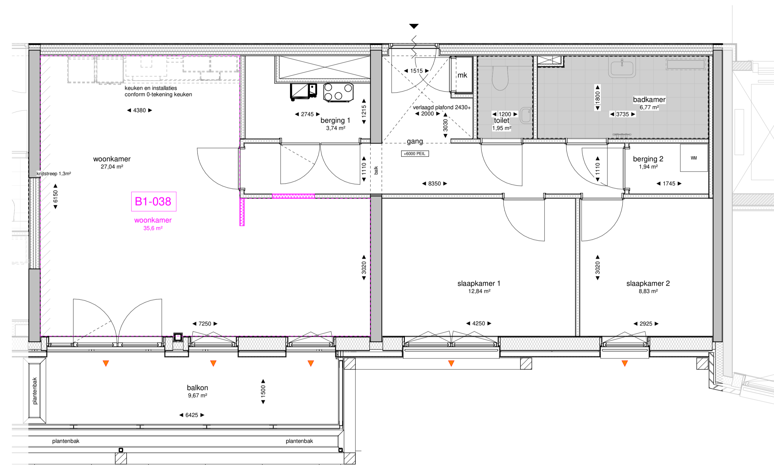
165-02 tweede verdieping optie schaal 1 : 50
