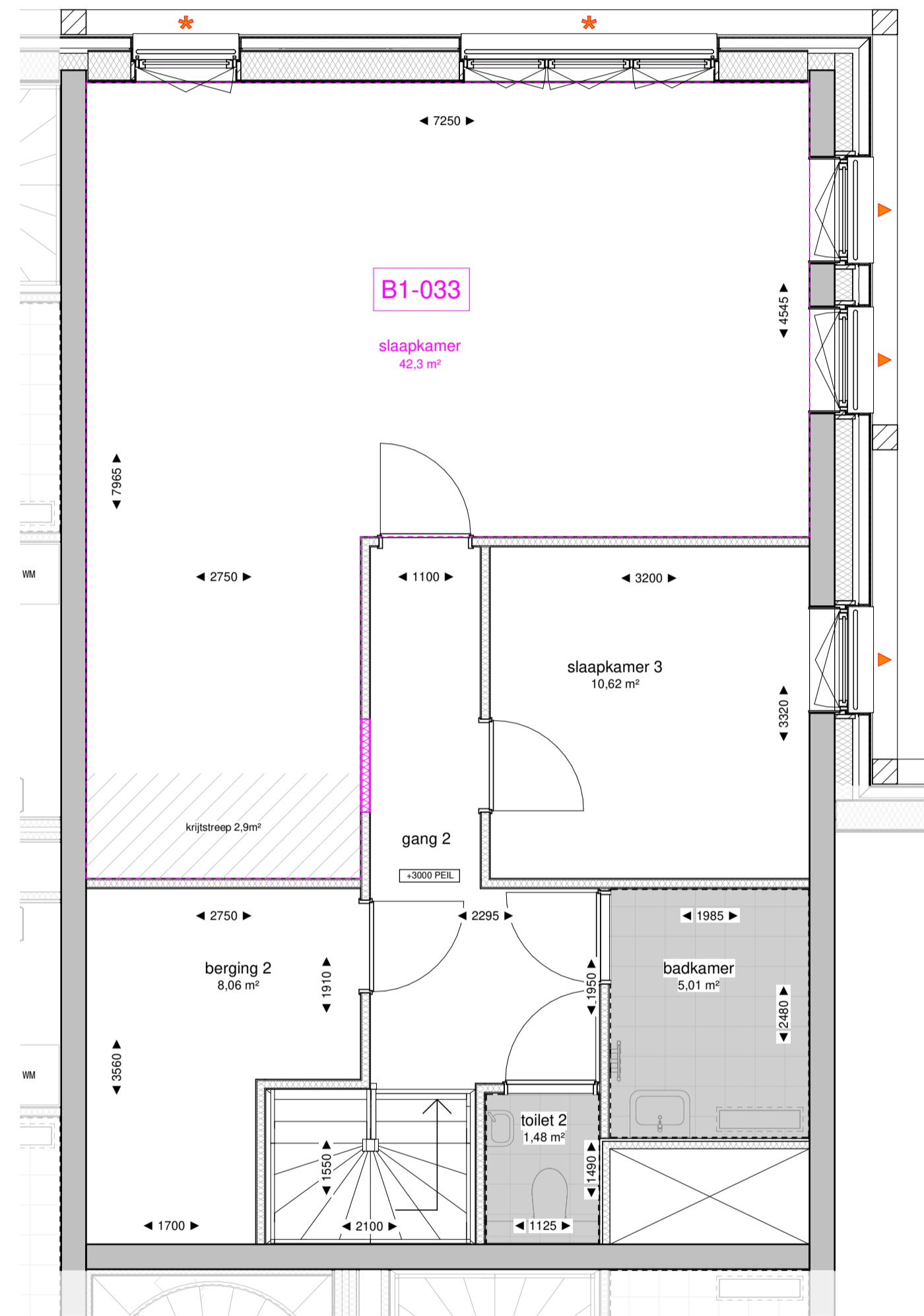
157-01 eerste verdieping optie schaal 1 : 50
