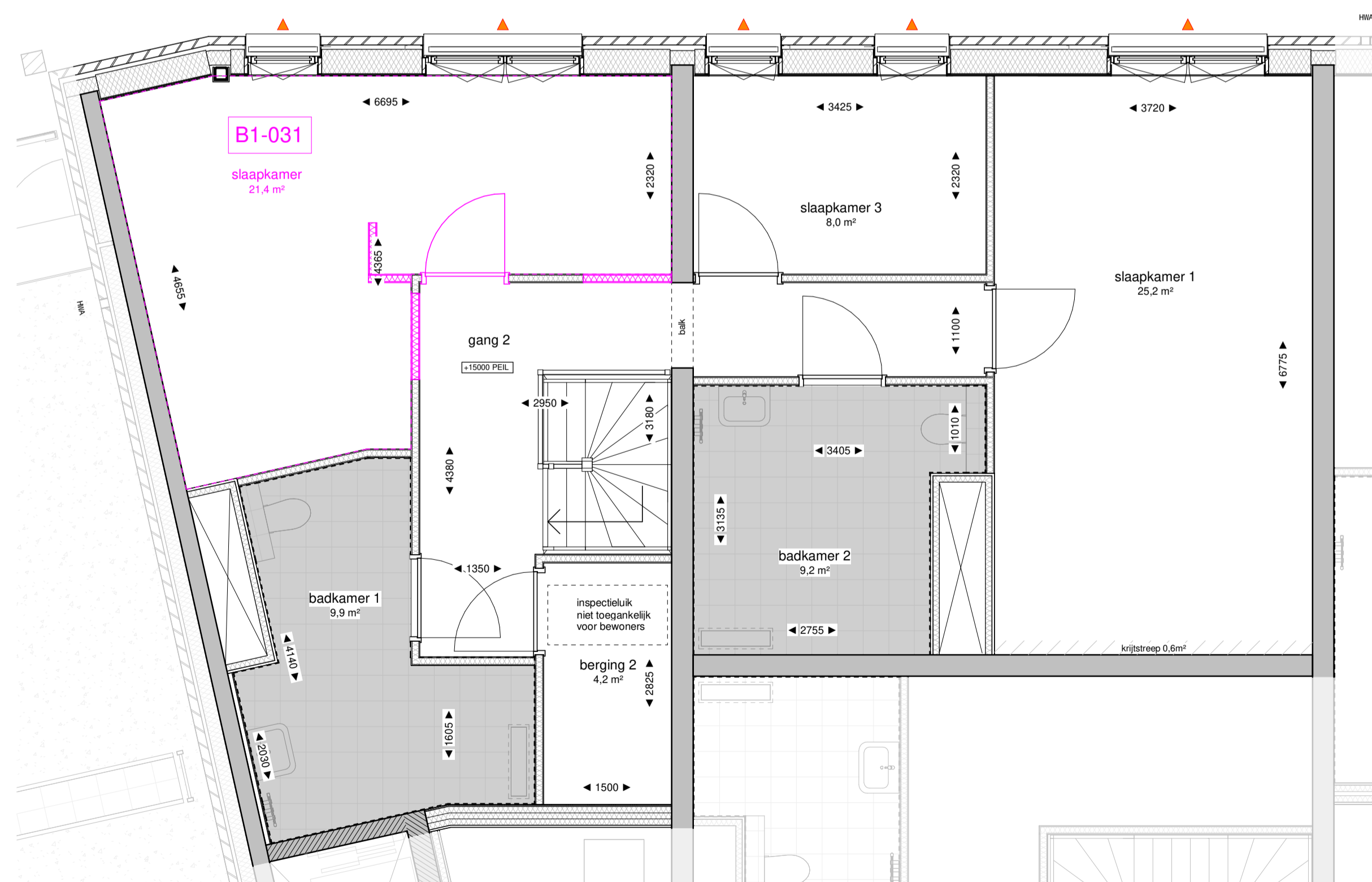
178-05 vijfde verdieping optie schaal 1 : 50
