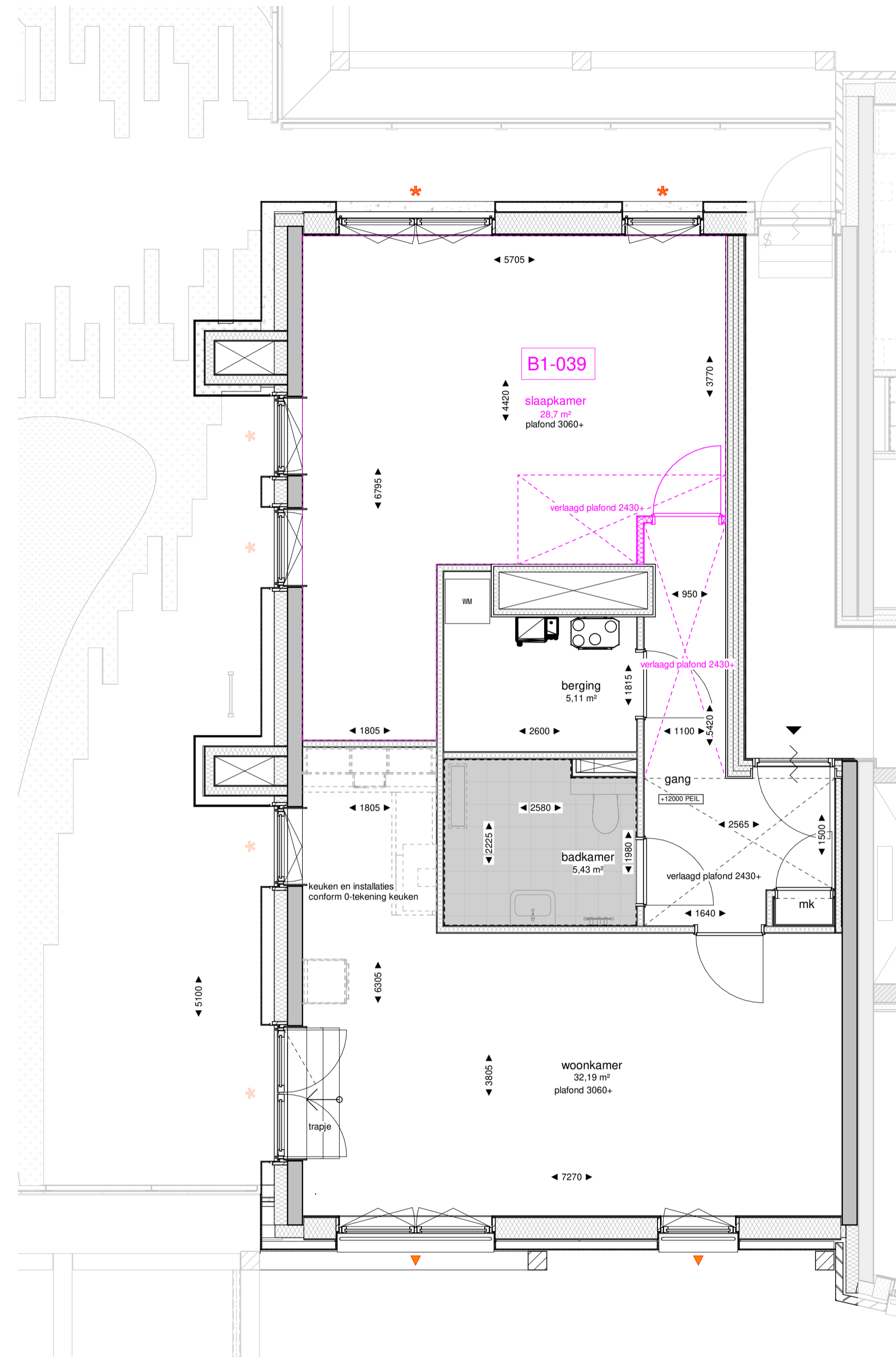
177-04 vierde verdieping optie schaal 1 : 50
