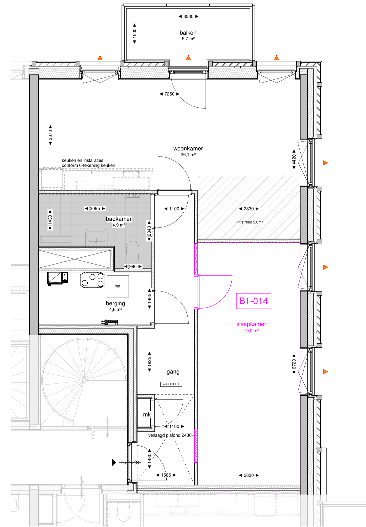
135-01 eerste verdieping optie schaal 1 : 50
