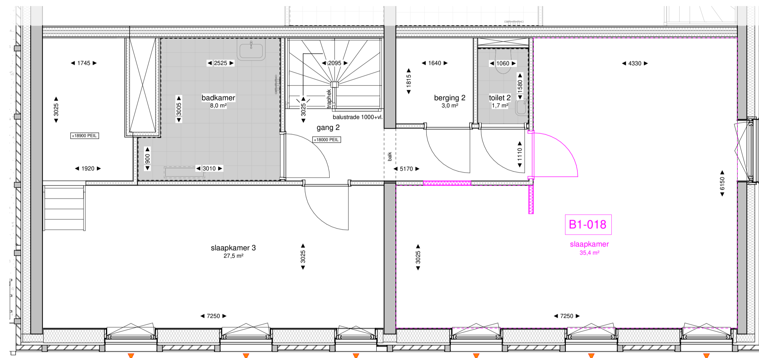
152-06 zesde verdieping optie schaal 1 : 50
