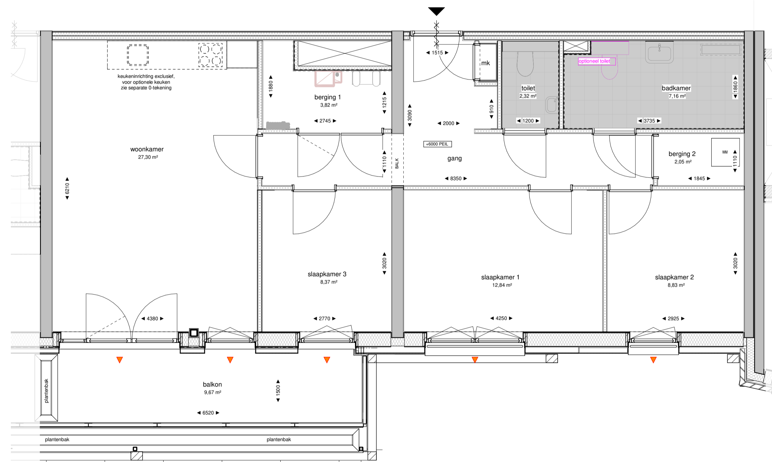
J.02.03 tweede verdieping optie schaal 1 : 50
