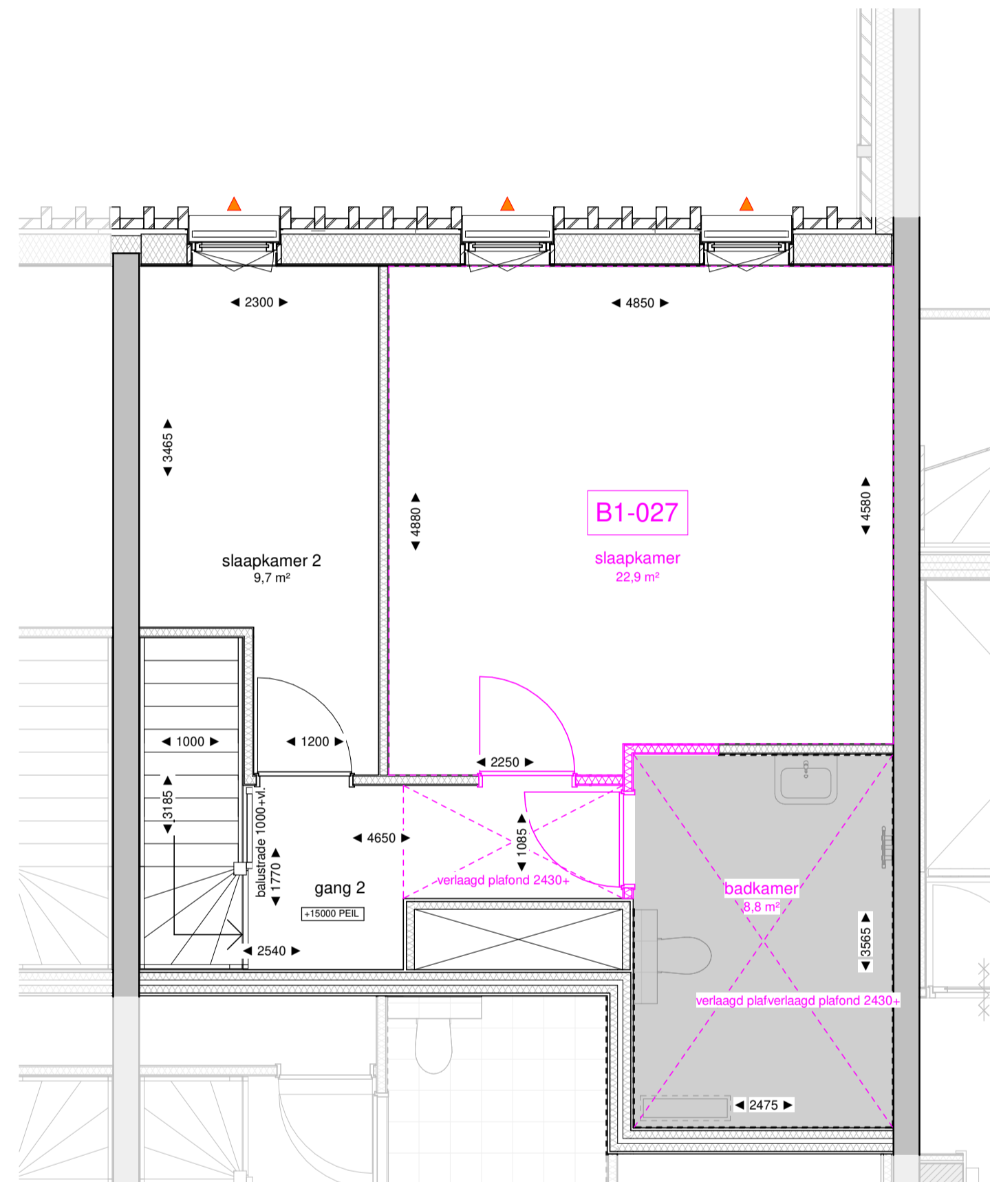
145-05 vijfde verdieping optie schaal 1 : 50
