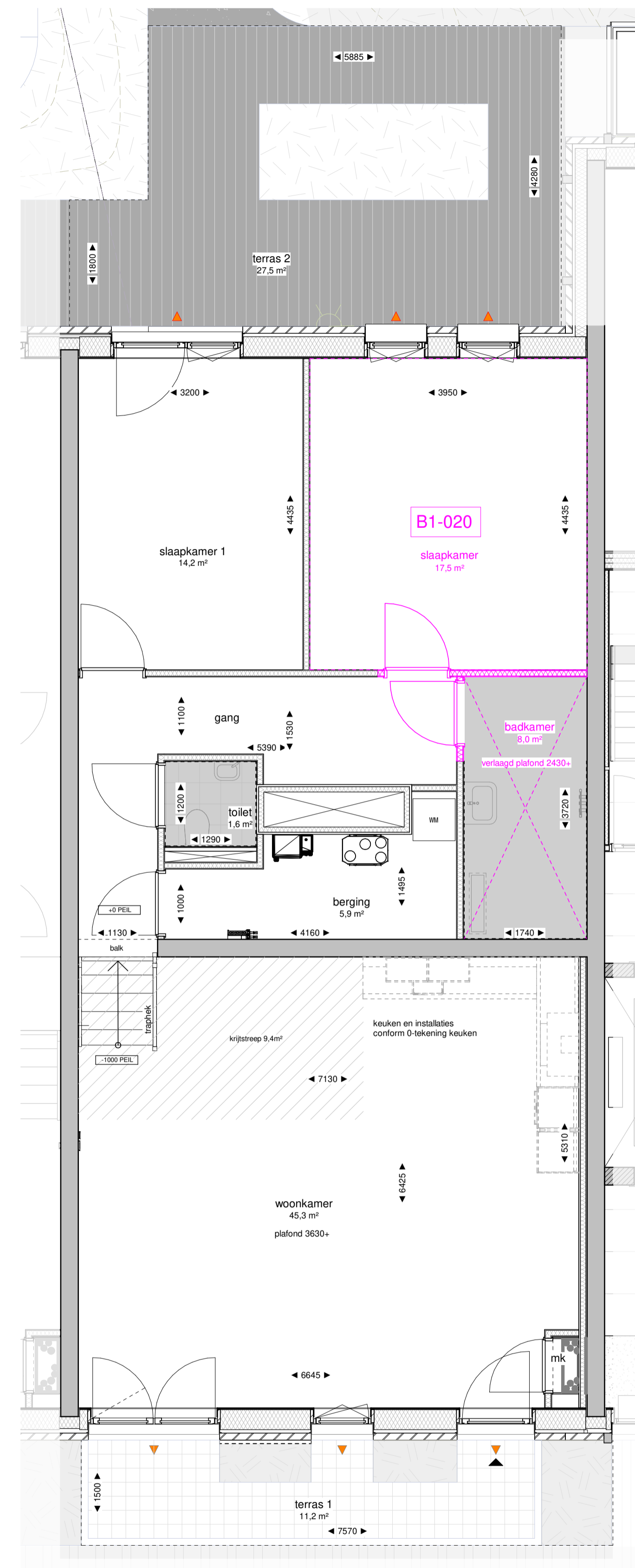
131-00 begane grond optie schaal 1 : 50
