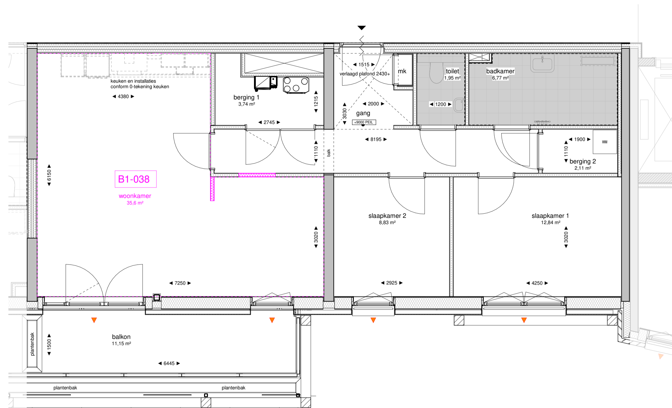
172-03 derde verdieping optie schaal 1 : 50
