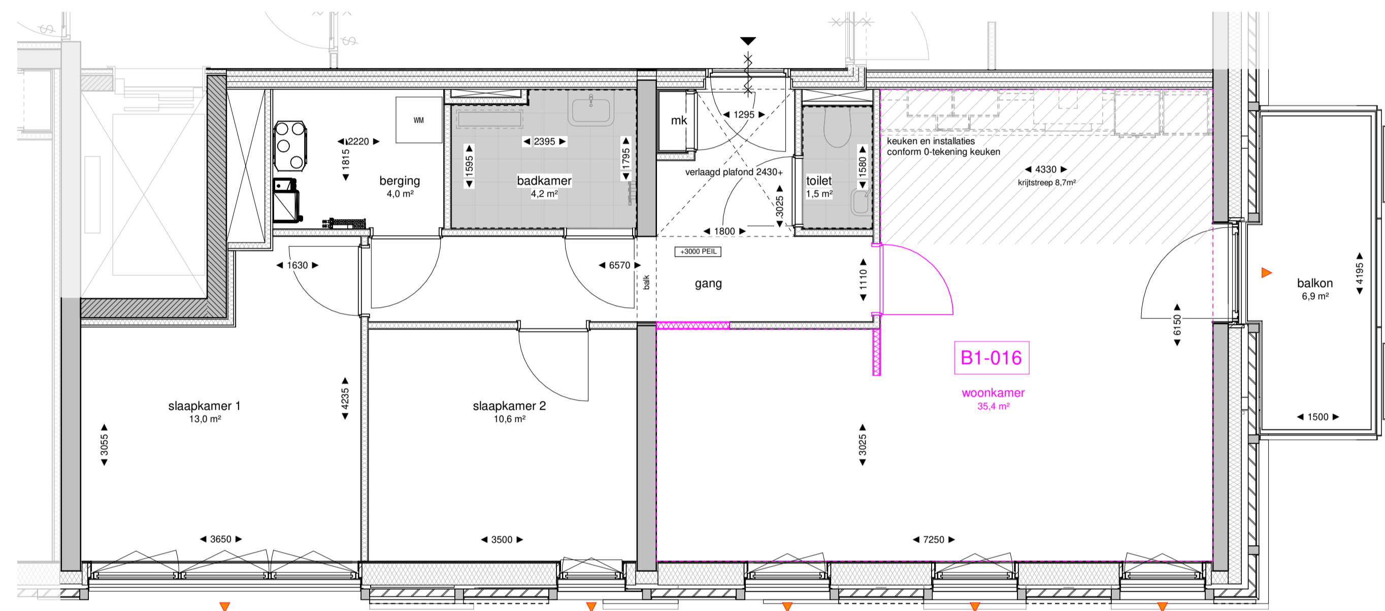
136-01 eerste verdieping optie schaal 1 : 50
