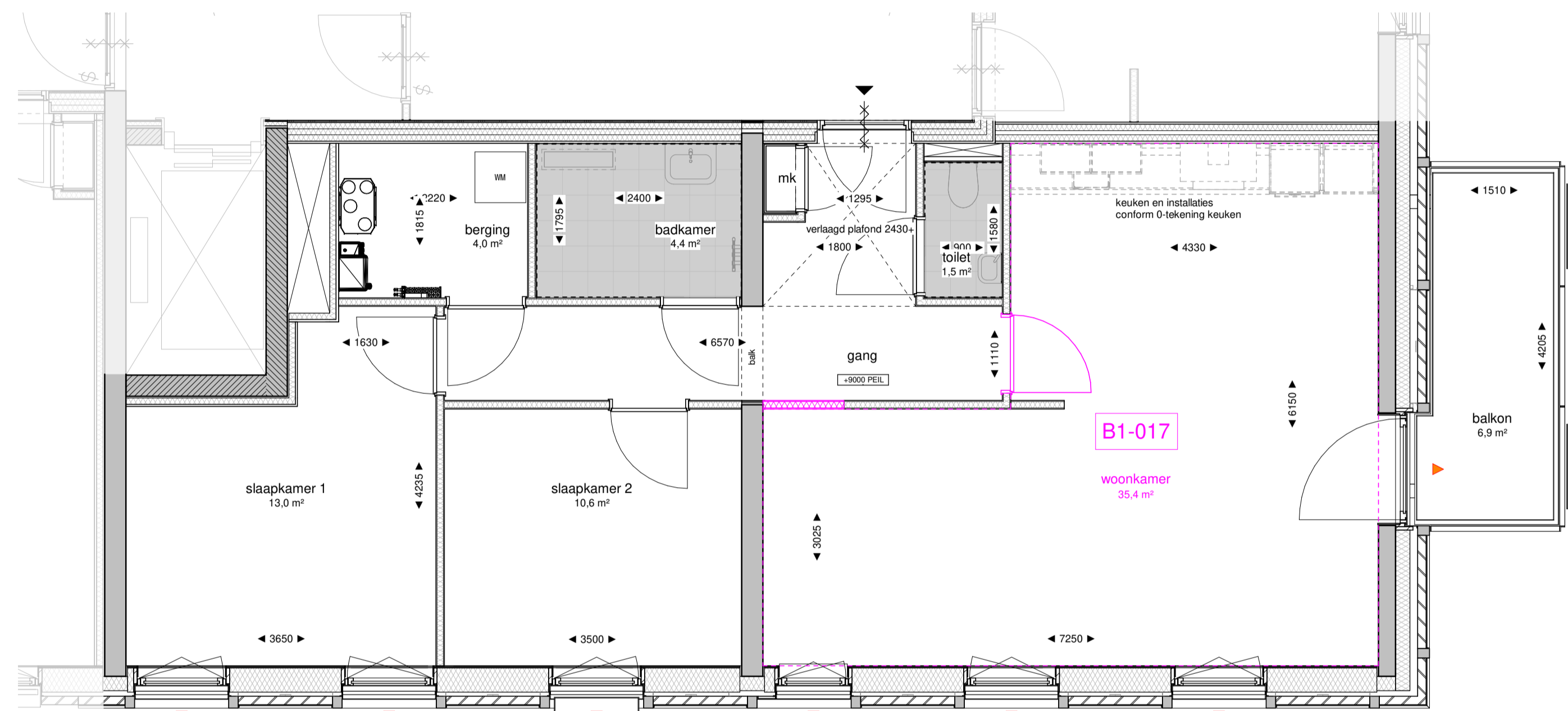
144-03 derde verdieping optie schaal 1 : 50
