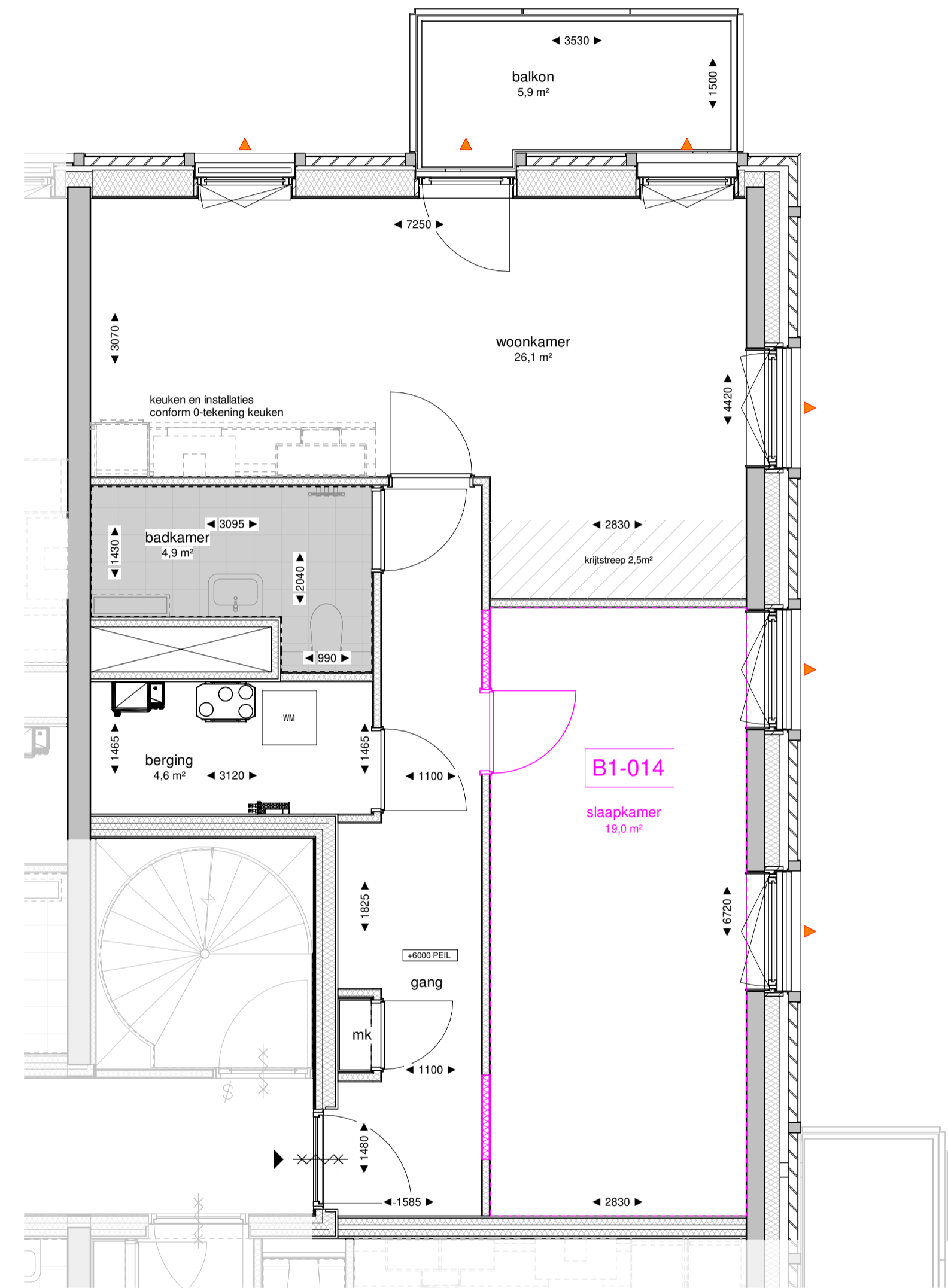
139-02 tweede verdieping optie schaal 1 : 50
