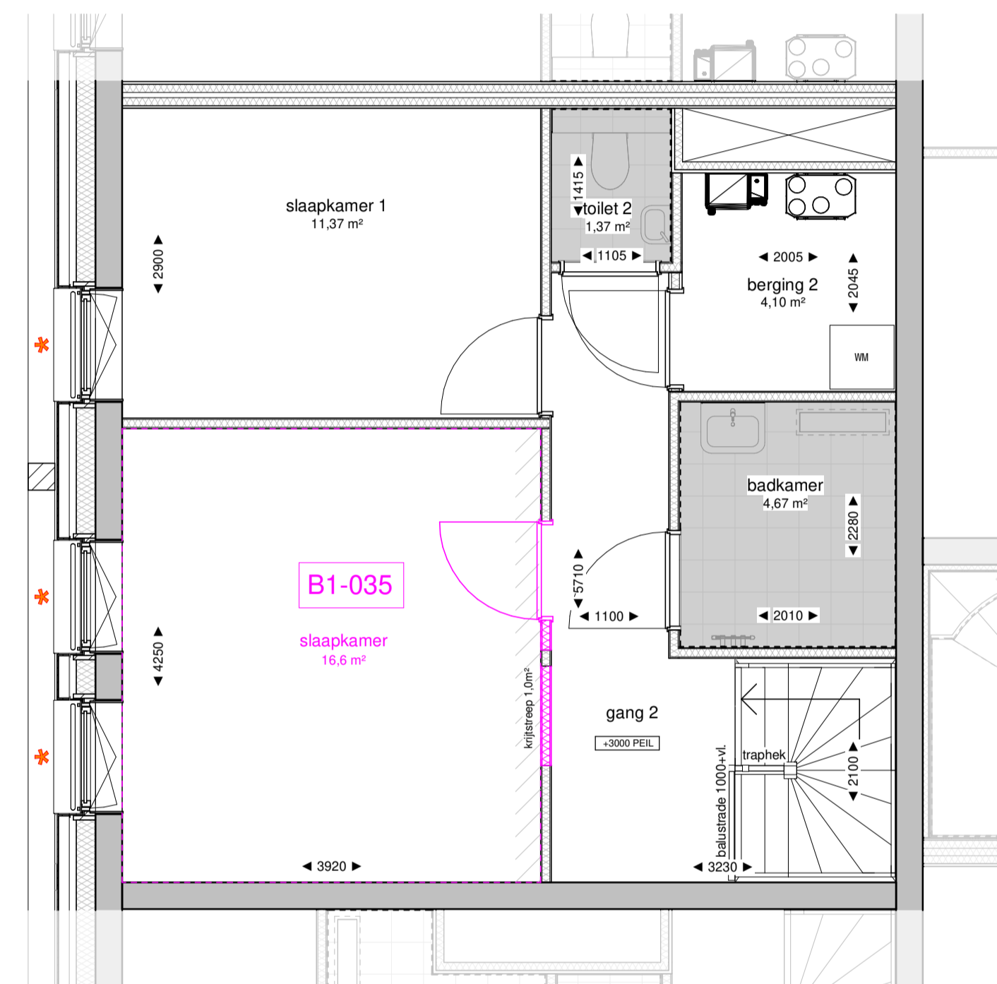
155-01 eerste verdieping optie schaal 1 : 50
