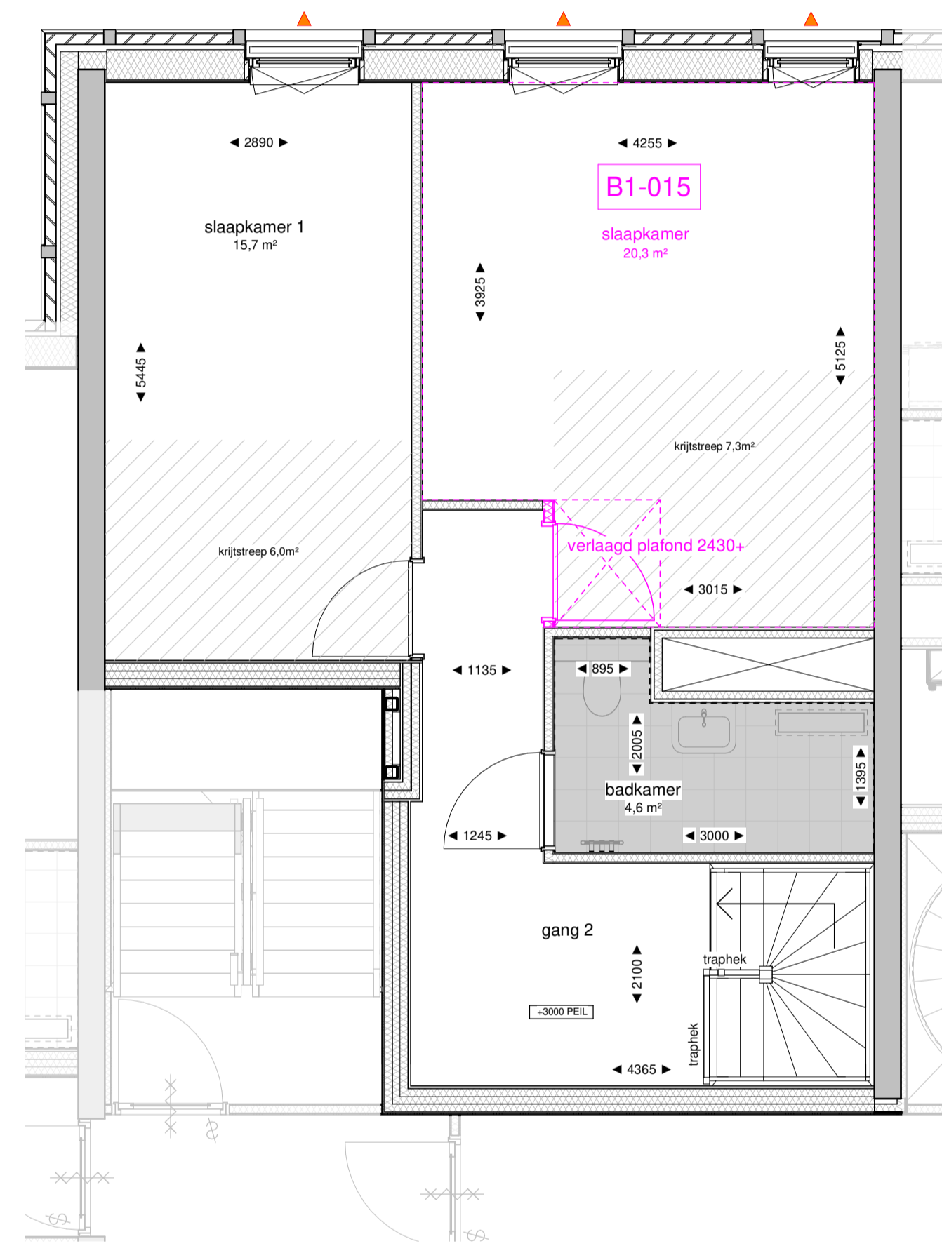
133-01 eerste verdieping optie schaal 1 : 50
