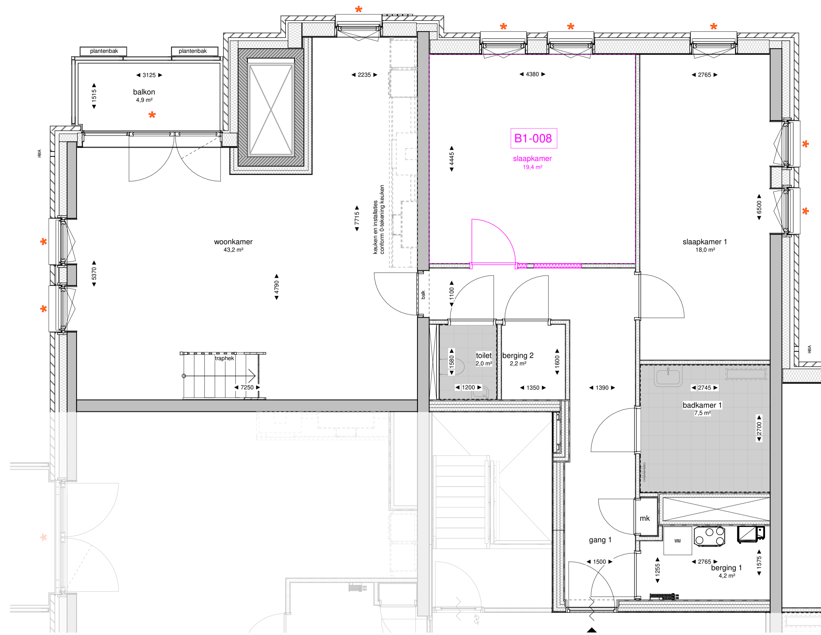
130-03 derde verdieping optie schaal 1 : 50
