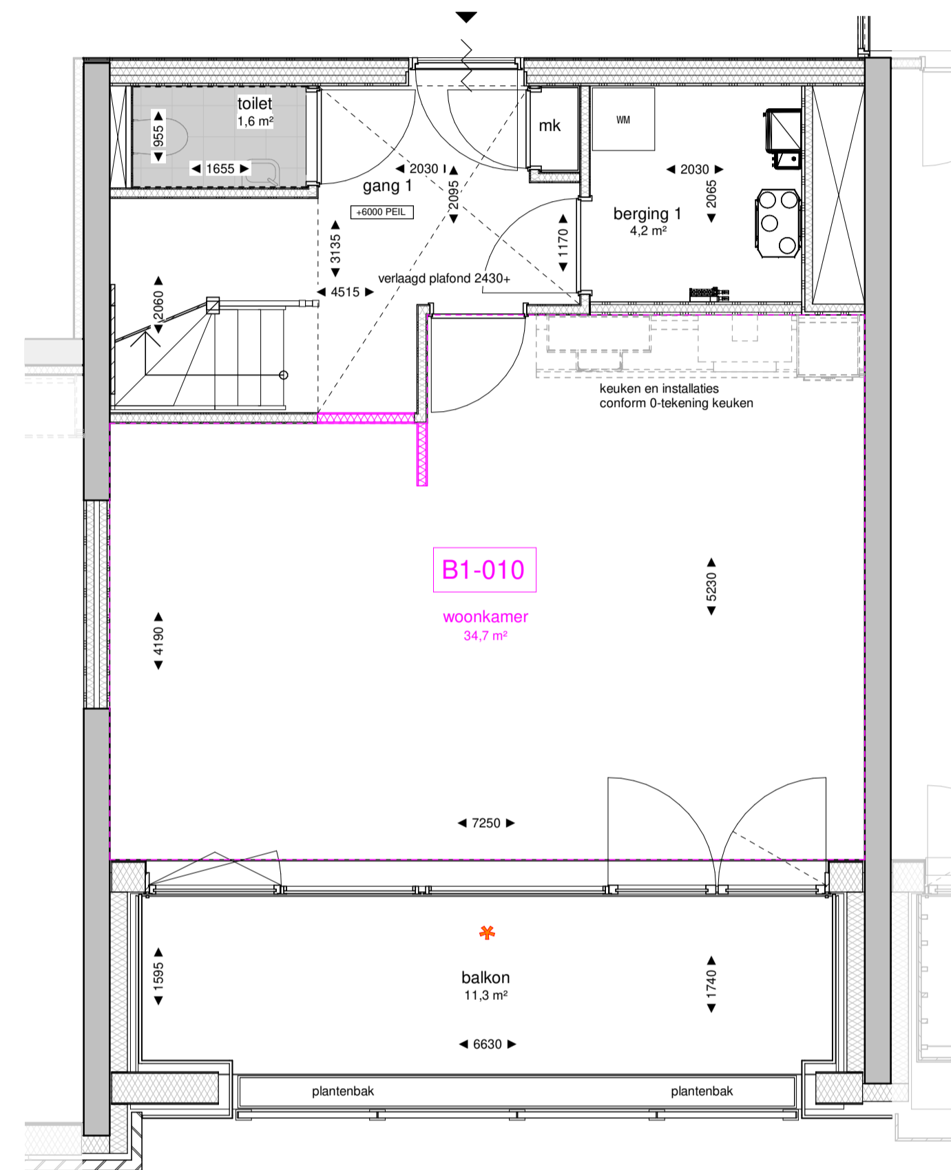
120-02 tweede verdieping optie schaal 1 : 50
