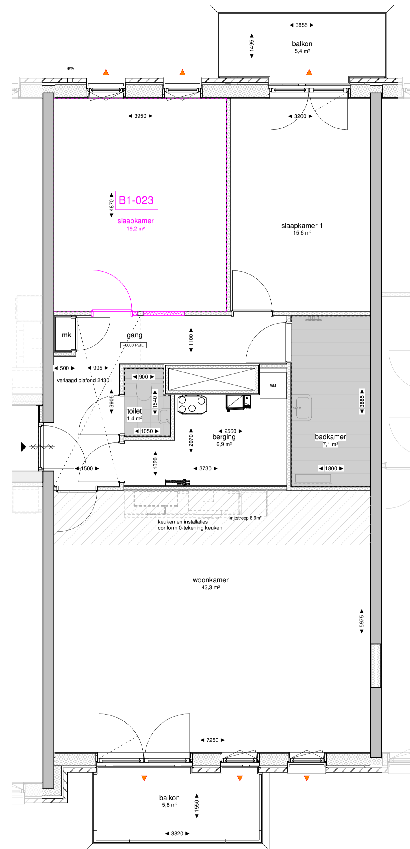
169-02 tweede verdieping optie schaal 1 : 50
