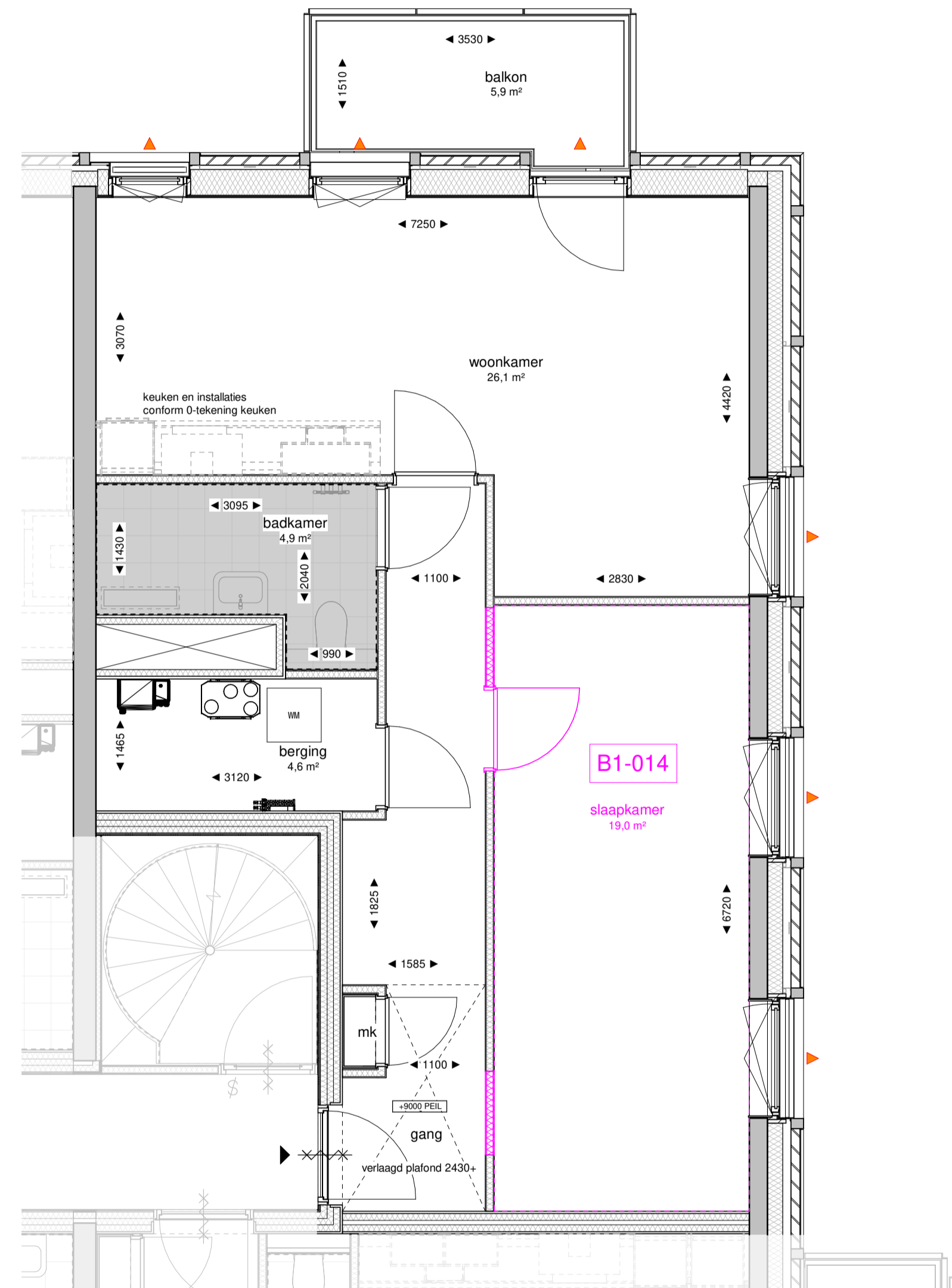
143-03 derde verdieping optie schaal 1 : 50
